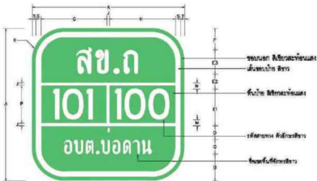
รูปที่ ข-๙ ตัวอย่างและรายละเอียดป้ายหมายเลขทางหลวงท้องถิ่น (น-๑/๑) ขนาด ๗๕x๗๕ ซม. (สำหรับ อปท. ลำดับที่ ๑๐๐- ๙๙๙)
