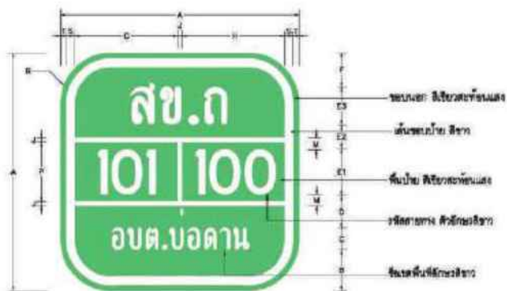
รูปที่ ข-๘ ตัวอย่างและรายละเอียดป้ายหมายเลขทางหลวงท้องถิ่น (น-๑/๑) ขนาด ๖๐x๖๐ ซม. (สำหรับ อปท. ลำดับที่ ๑๐๐ - ๙๙๙)
